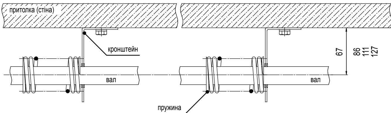
ВАРІАНТ КРІПЛЕННЯ ДВОХ ЛІВИХ ПРУЖИН
