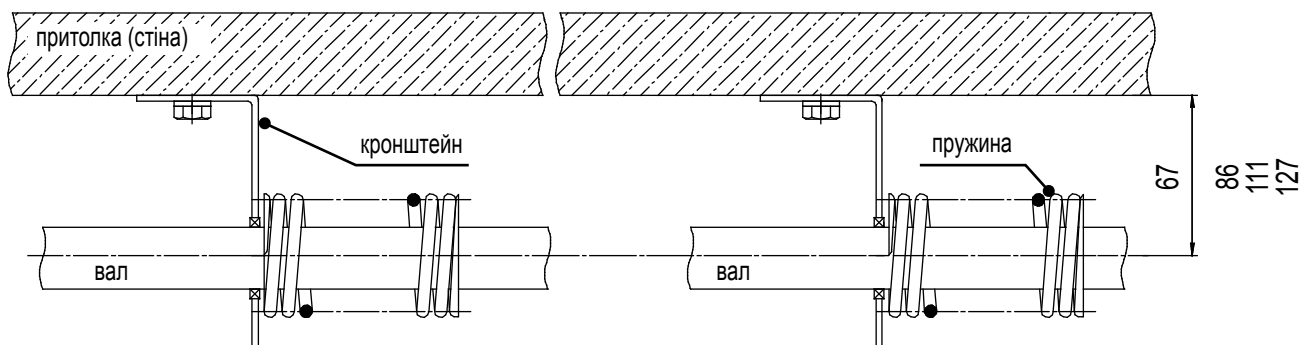
ВАРІАНТ КРІПЛЕННЯ ДВОХ ПРАВИХ ПРУЖИН ІЗ ЗАХИСТОМ ВІД РОЗРИВУ ПРУЖИН
