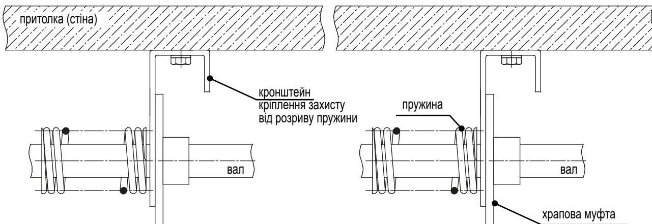
ВАРІАНТ КРІПЛЕННЯ ДВОХ ЛІВИХ ПРУЖИН ІЗ ЗАХИСТОМ ВІД РОЗРИВУ ПРУЖИН
