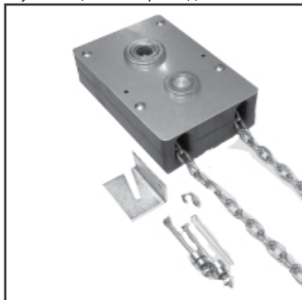
Ручной цепной привод
